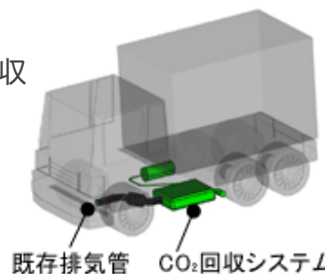
【車載式CO 2 回収システム】
