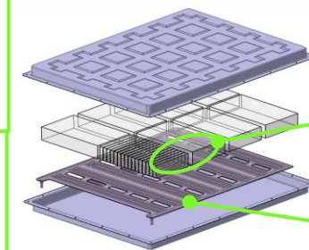
【バッテリー冷却プレート】
